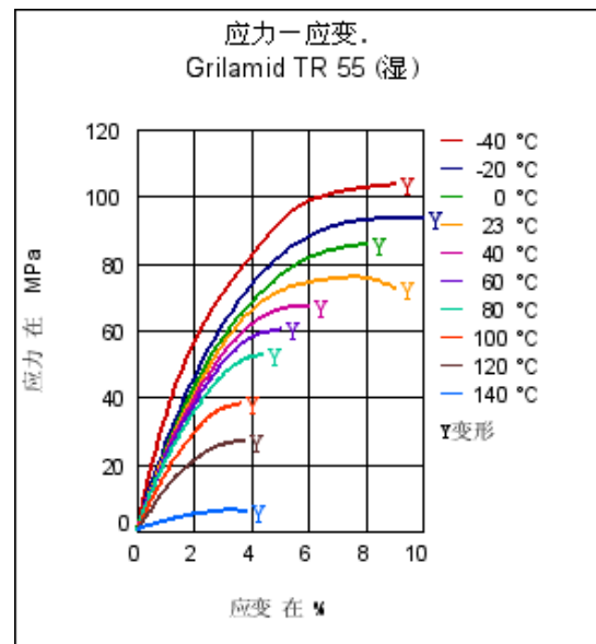
应力 - 应变
